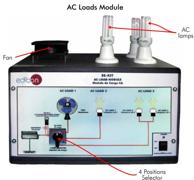
AC Loads Module
